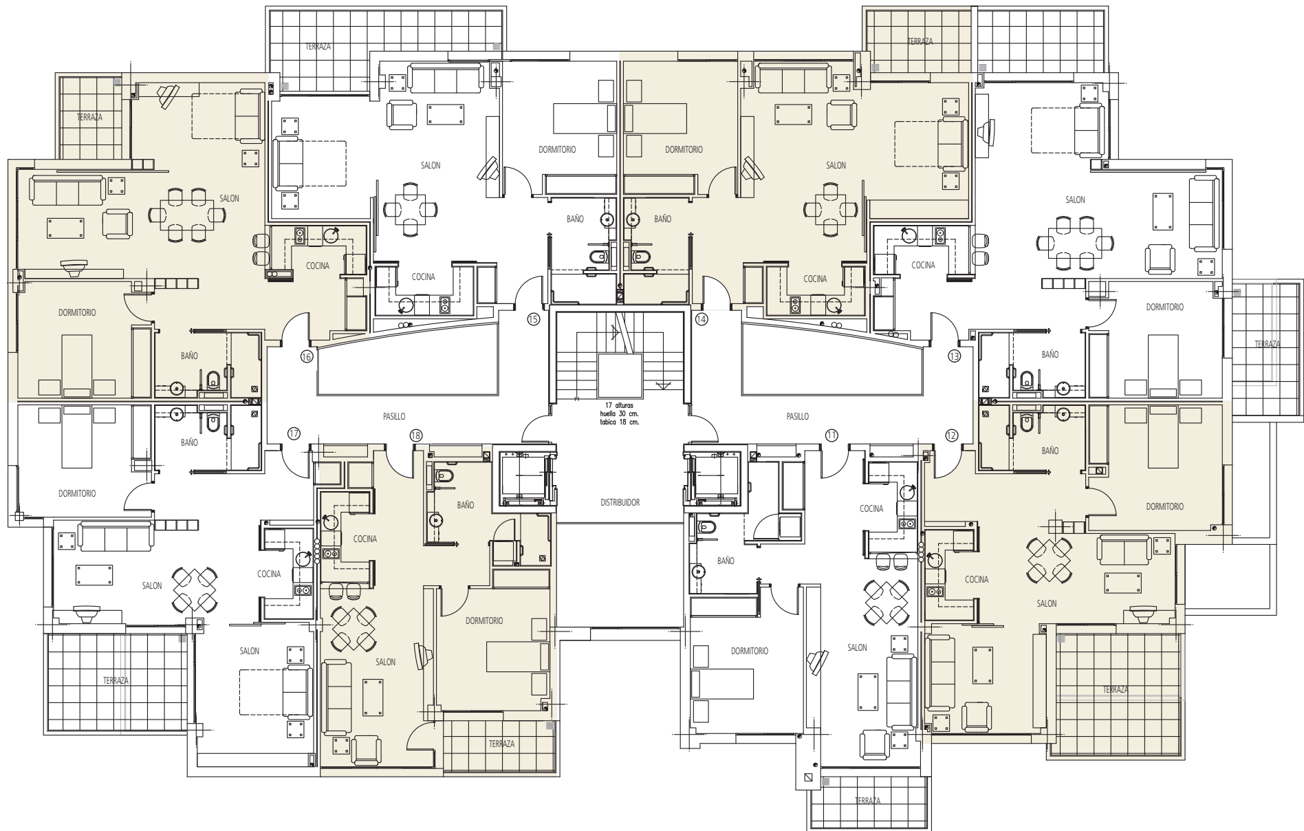
PLANTA PRIMERA
