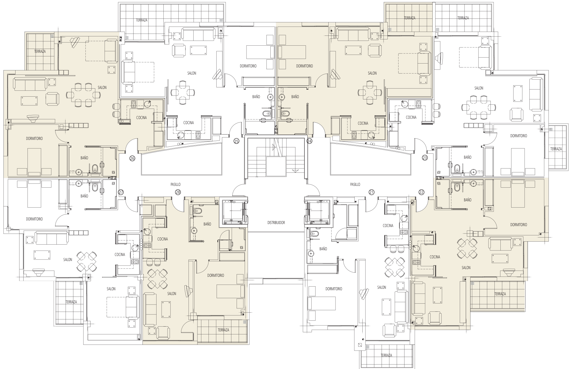
PLANTA SEGUNDA
